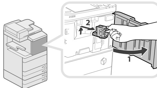
Unidad de Acabado Interna E1 (Opcional)
