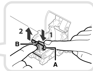
Sattelhefteinheit des Broschüren Finisher J1
